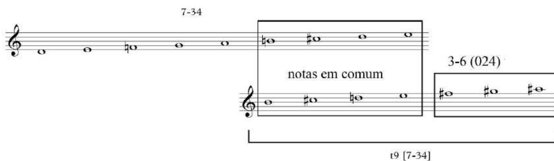
Figura 33 – classes de notas em comum entre 7-34 e t_9[7-34]
